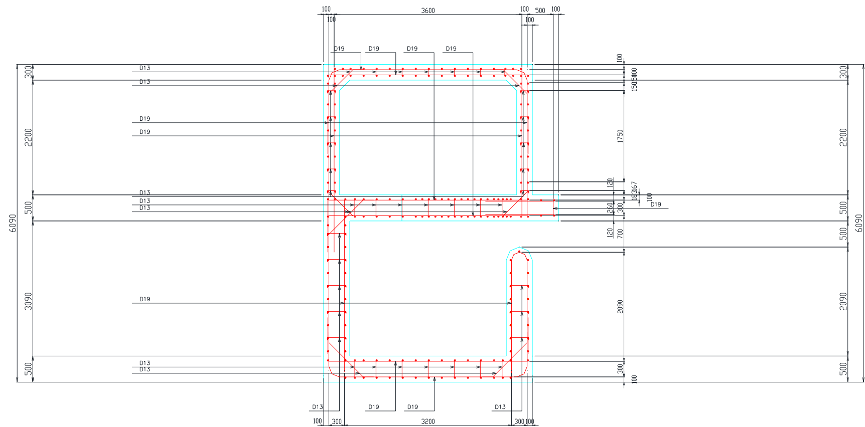
沈砂池配筋図の一例
